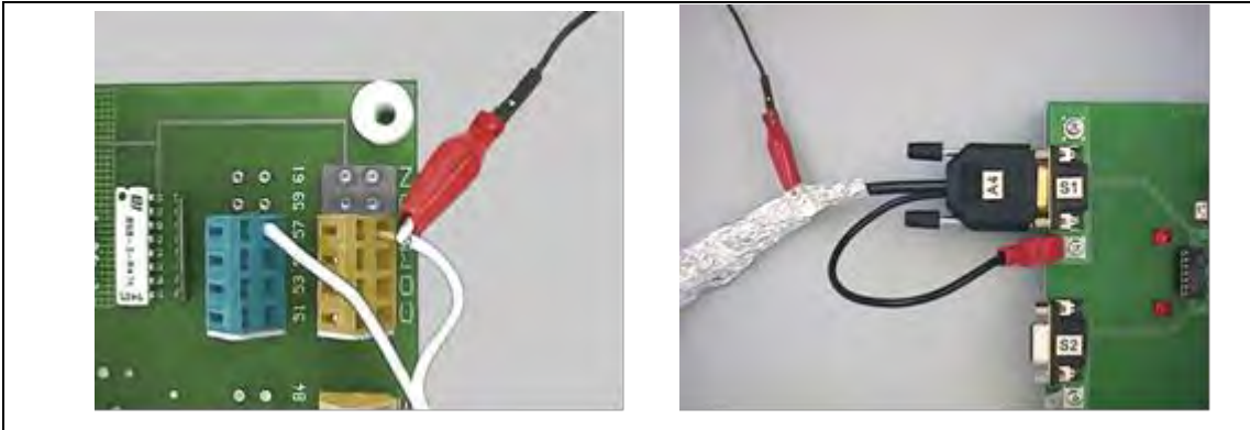
图 23: 发生器直接连接到控制和辅助电源线。与数据线中，发生器的极被连接到线屏蔽或电容器涂层
