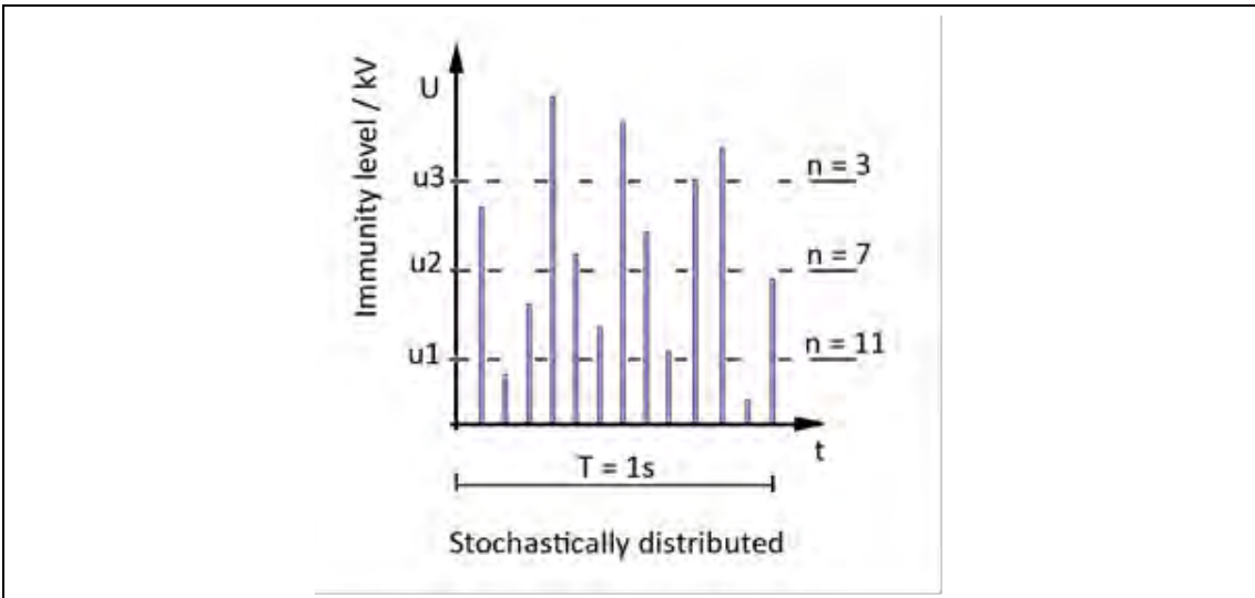
图 16: 该 SGZ 21 以无序的方式连续生成脉冲
