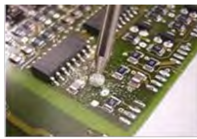
图 28：通过点朝向准备地层，焊接接触引脚，发生器电缆用微型探针连接到接触引脚，经由导体注入干扰电流到地。
