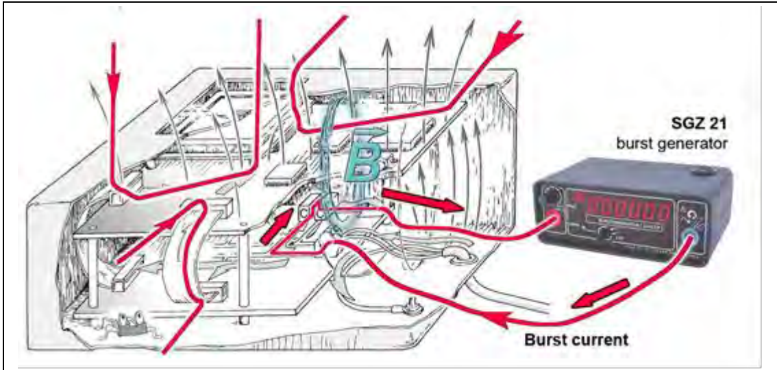
图 19: 用 SGZ 21 二极管注入到被测设备。
