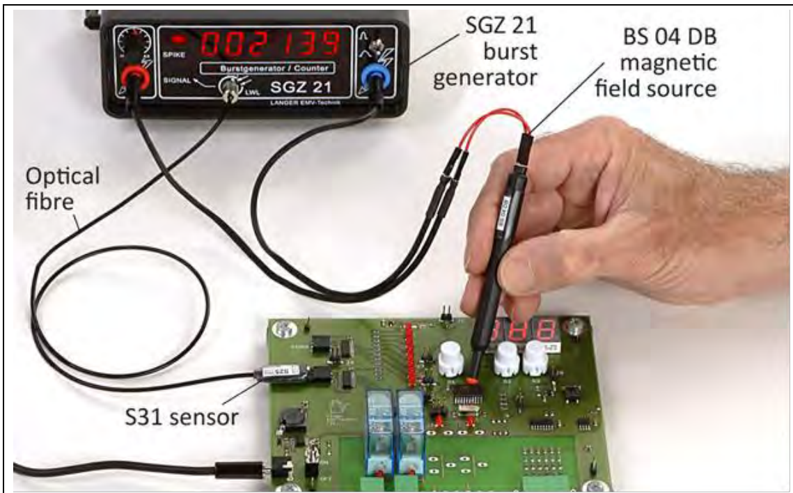
图 38: 磁场源跨过模块引导到直接应用的磁场导体环路
