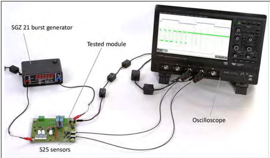
图 50: 测试设置有两个通道的光信号的采集来产生被测设备干扰的波形图。
