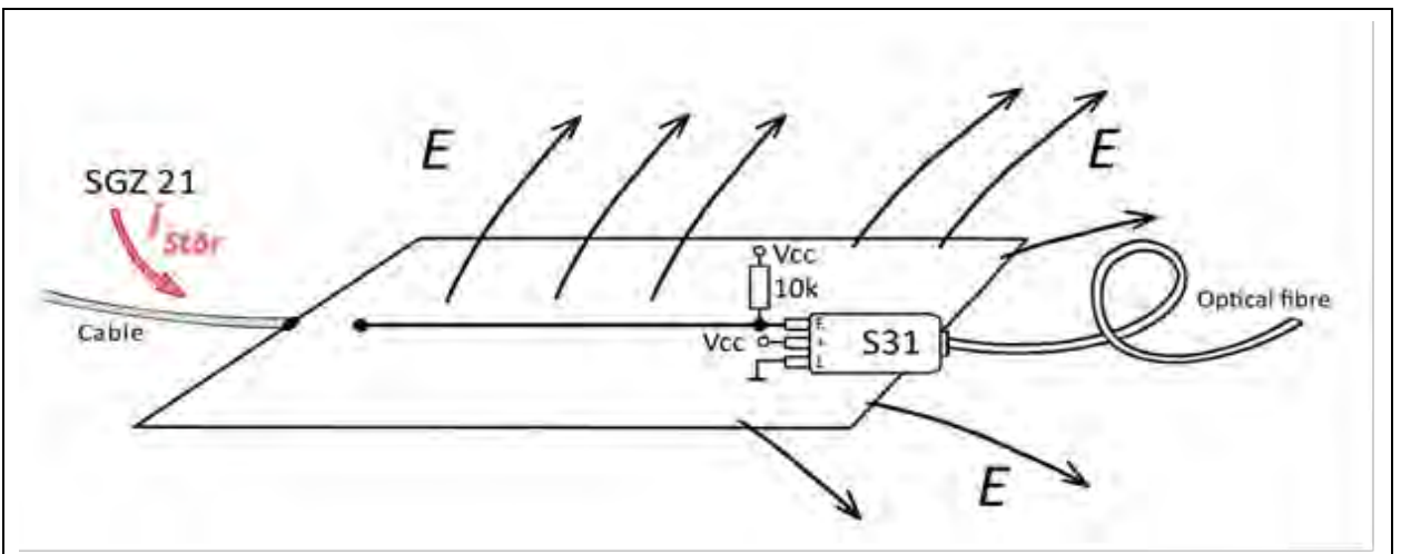
图 14: 通过安装与漆包铜线的 S31 传感器作为模拟导体段建立人工电场抗干扰等级
