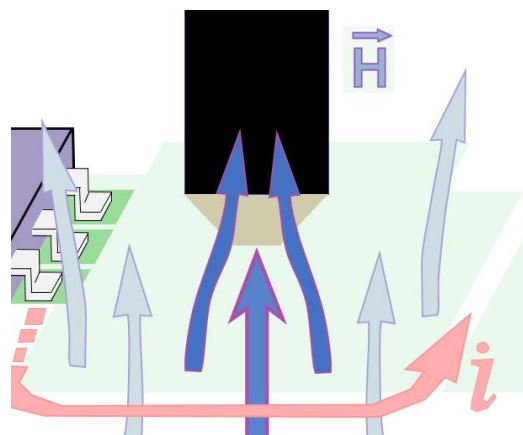
图 2 OI-ICH40 磁场探头捕获信号路径
