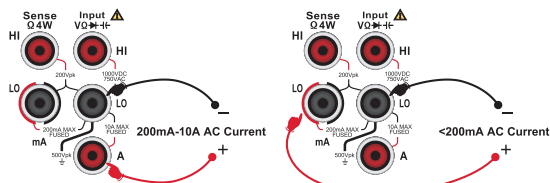
图2-12交流电流测量连接示意图
