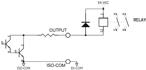
图9-2-6-1 控制继电器
