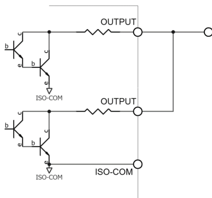
图9-2-6-4双端口输出组成逻辑或电路
