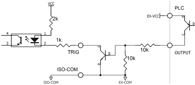
图9-2-5-4使用PLC正公共端子控制
