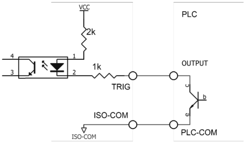
图9-2-5-3使用PLC负公共端子控制
