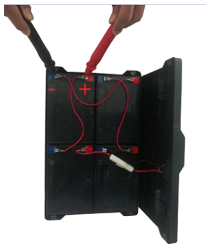
图3-3-2皇冠探头测试笔测量示意图
