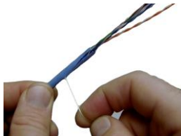
拉动尼龙线绳，保证中心导体无缺口
